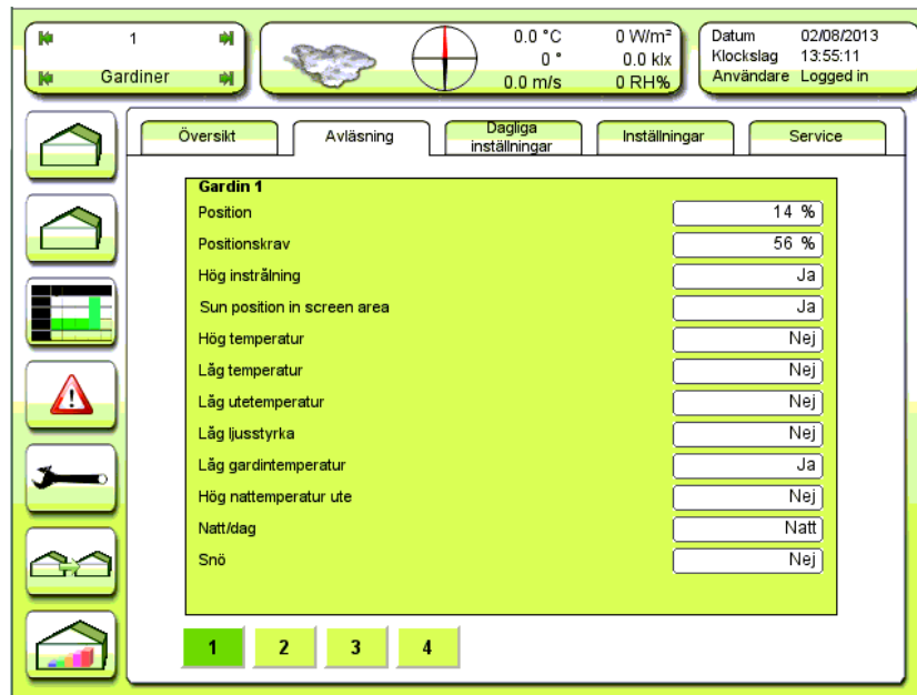
Figur 28 Avläsning av status för gardin 1.
