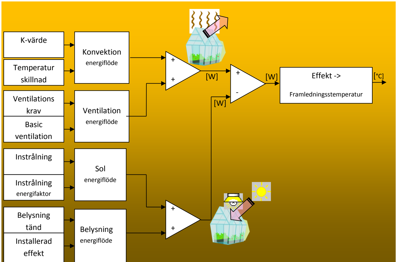
Figur 95 Energibalansmodellen
