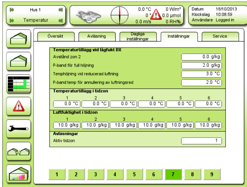
Figur 120 Temperaturlägg vid lågfukt enligt Delta X
